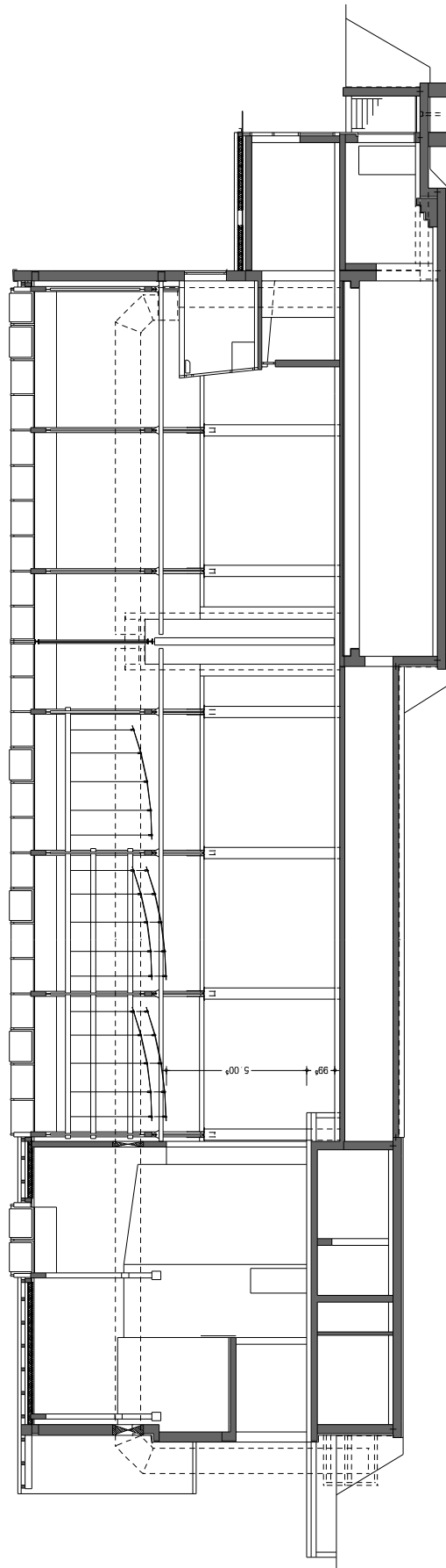
SCHNITT BÜRGERSAAL/BÜHNE
